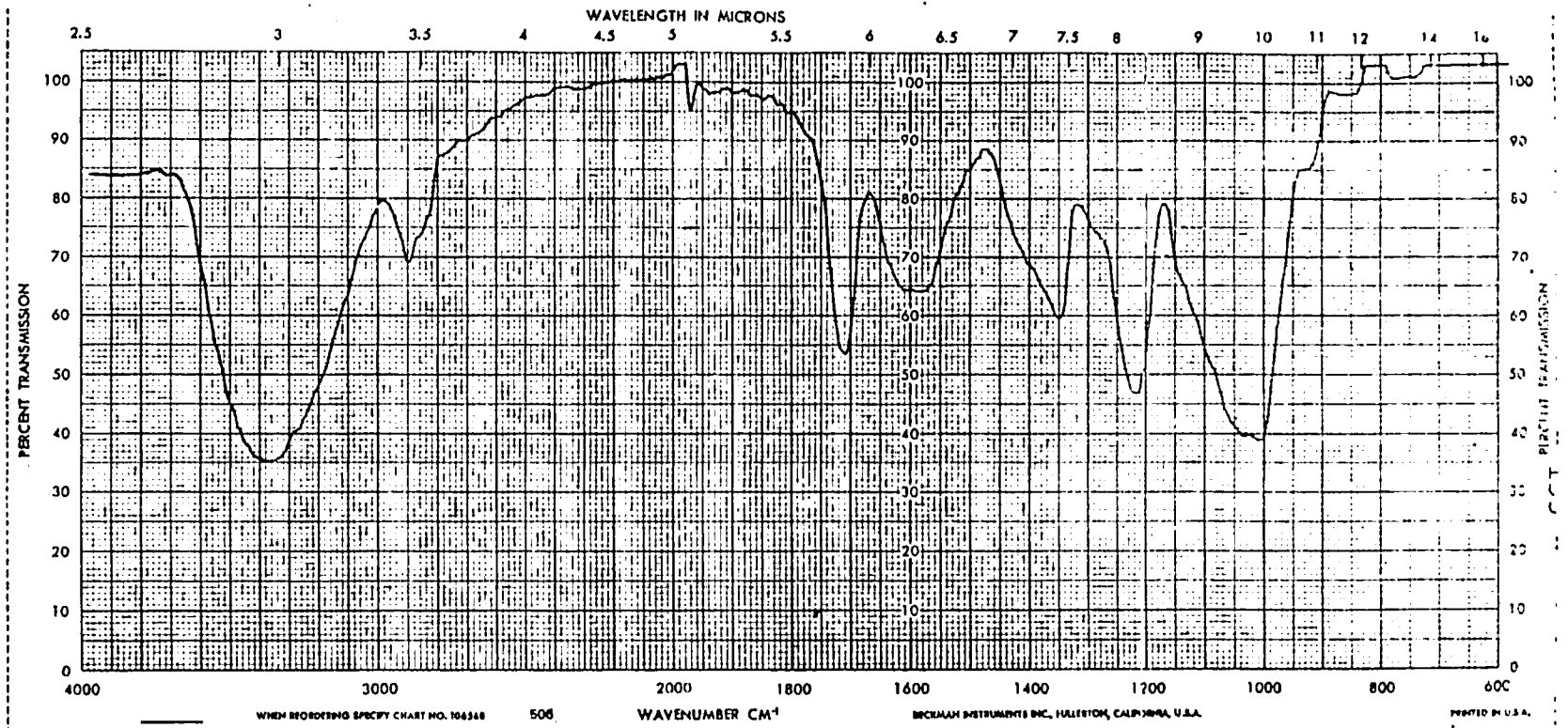
FIGURA 11. ESPECTRO INFRARROJO DEL CONCENTRADO 1.-
